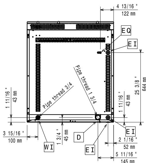
Boven aanzicht
